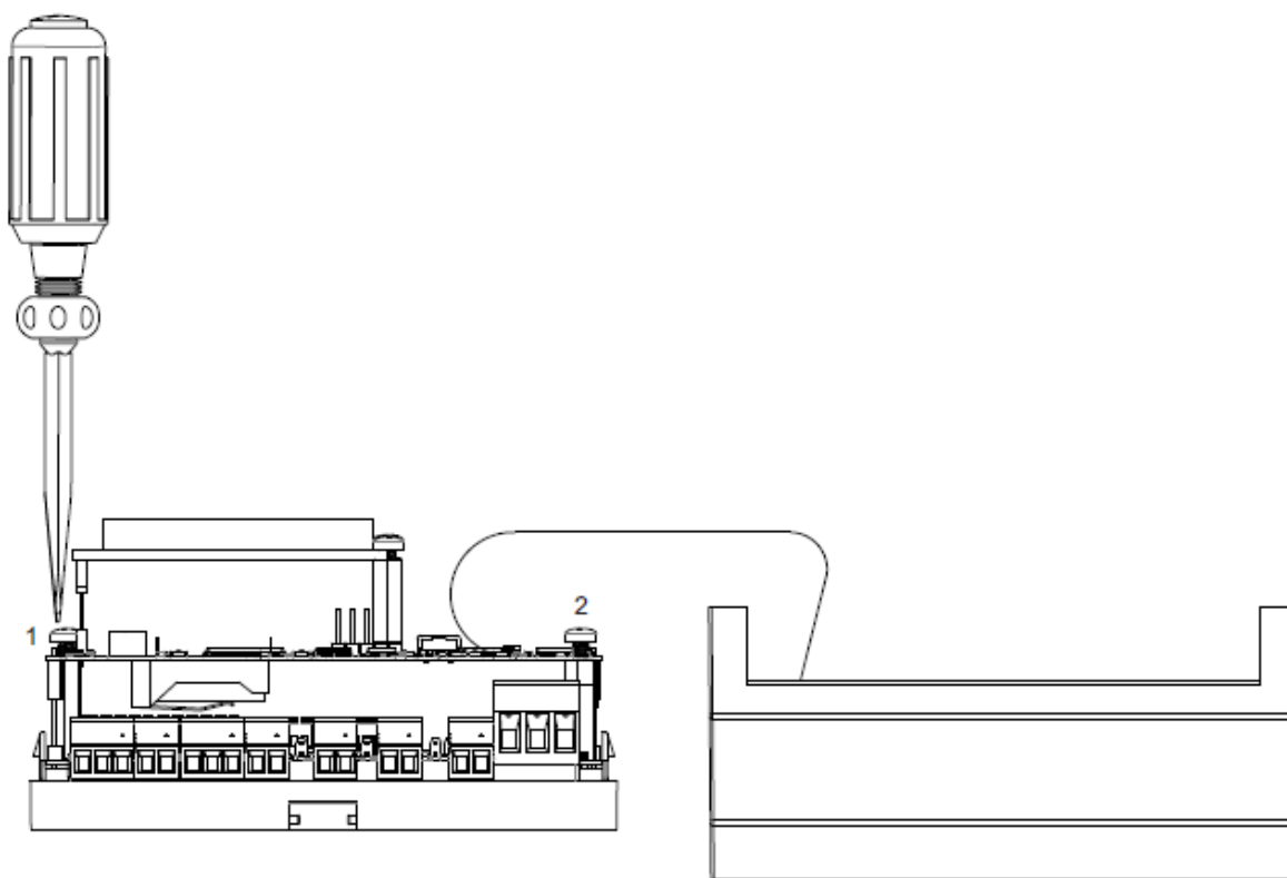
Рисунок 29 – Откручивание винтов
